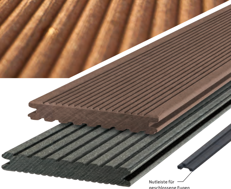
Abbildung zeigt CLASSIC 21 x 145 mm, feingeriffelt, mit offener Fuge, in Naturbraun
