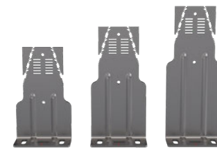
EQUERRE MURALE Matériau : aluminium DS 140 - 160 (Longueur 187,5 mm) DS 180 - 200 (Longueur 227,5 mm) DS 220 - 240 (Longueur 267,5 mm)
