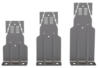
WALL BRACKET Material: Aluminium DS 140 - 160 (Length 187,5 mm) DS 180 - 200 (Length 227,5 mm) DS 220 - 240 (Length 267,5 mm)
